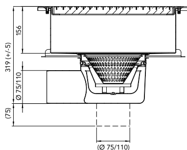
SEKTION A-A
