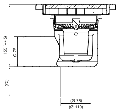
SEKTION A-A
