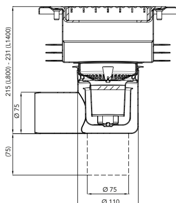
SEKTION A-A
