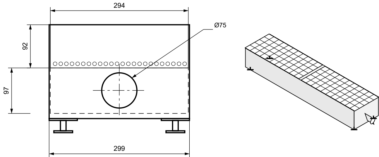
ISOMETRISK VY – ej skalenlig
