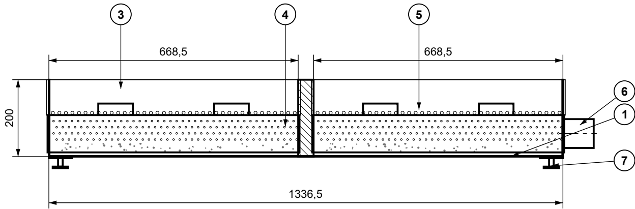
SNITT A–A SECTION A–A (1:10) Höjden 200 mm avser lådan. Ställbenen tillkommer.
