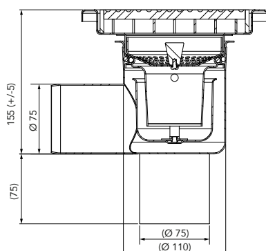
SEKTION A-A
