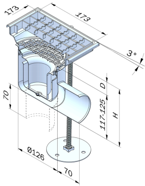
Mått för golvbrunn FURO 104
