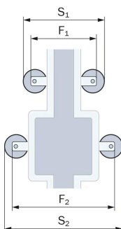
Byggmått för golvränna FURO 164:
