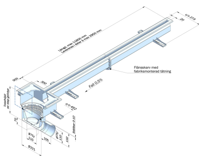
Mått för golvränna FURO 164
