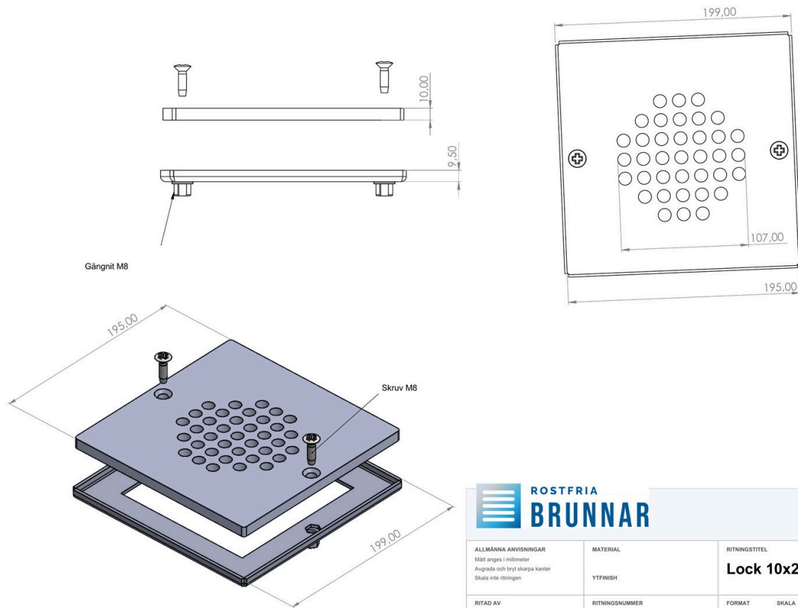
Klinkerram Industri 200x200mm – galler med ram, skruv M8 och gängnit M8. Mått i mm.
