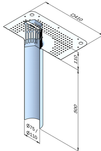
FURO180 Måttskiss
