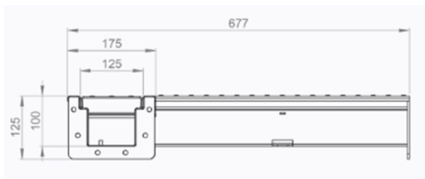
Måttskiss DRYLINE Modul 90° och T
