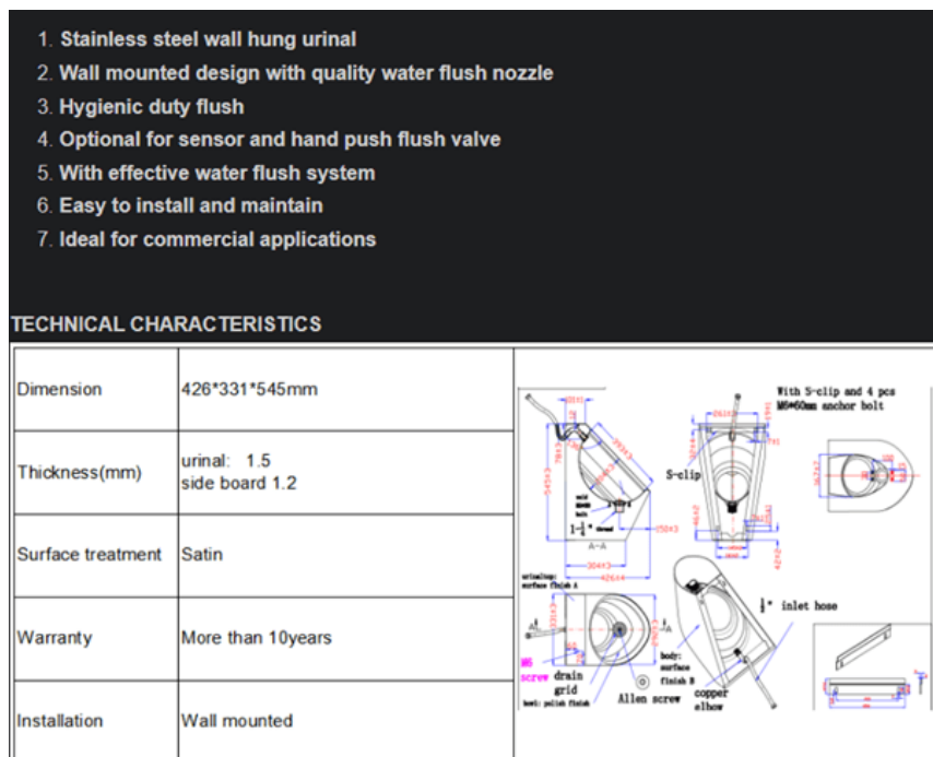
Måttskiss Piss1 Urinal
